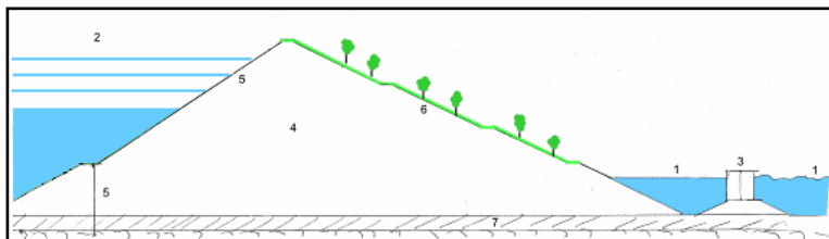
Coupe d'un atoll de stockage d'énergie
